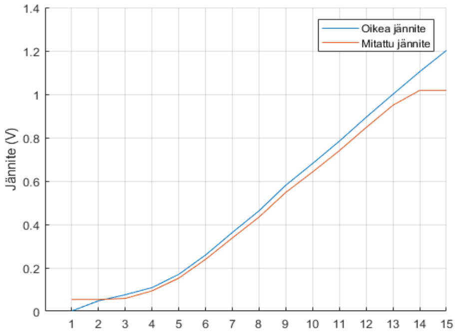
kuva 15. SiPyn sisäisen A/D-muuntimen mitaaman jännitteen ja syötetyn jännitteen kuvaajat
