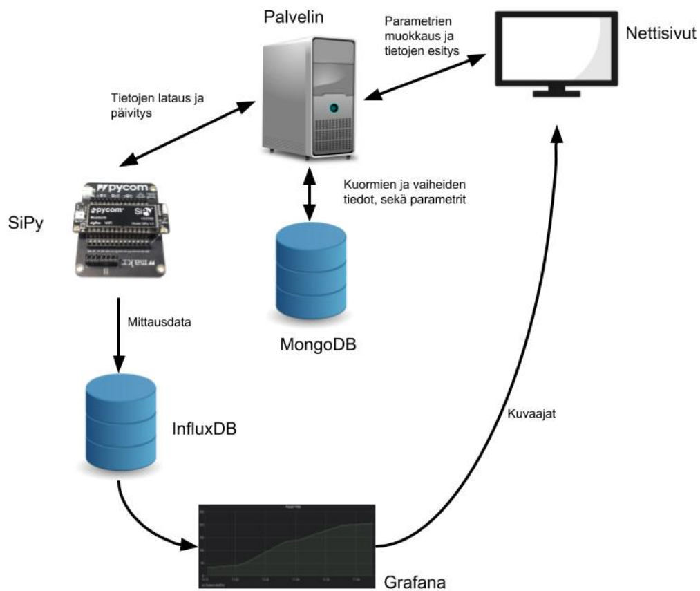
kuva 19. Ohjelmiston ja tietokantojen väliset riippuvuudet.
