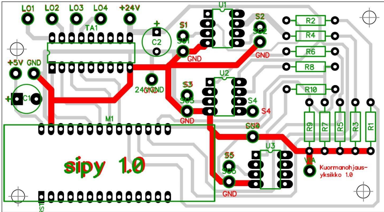
kuva 1. Piirilevyn suunnitelma
