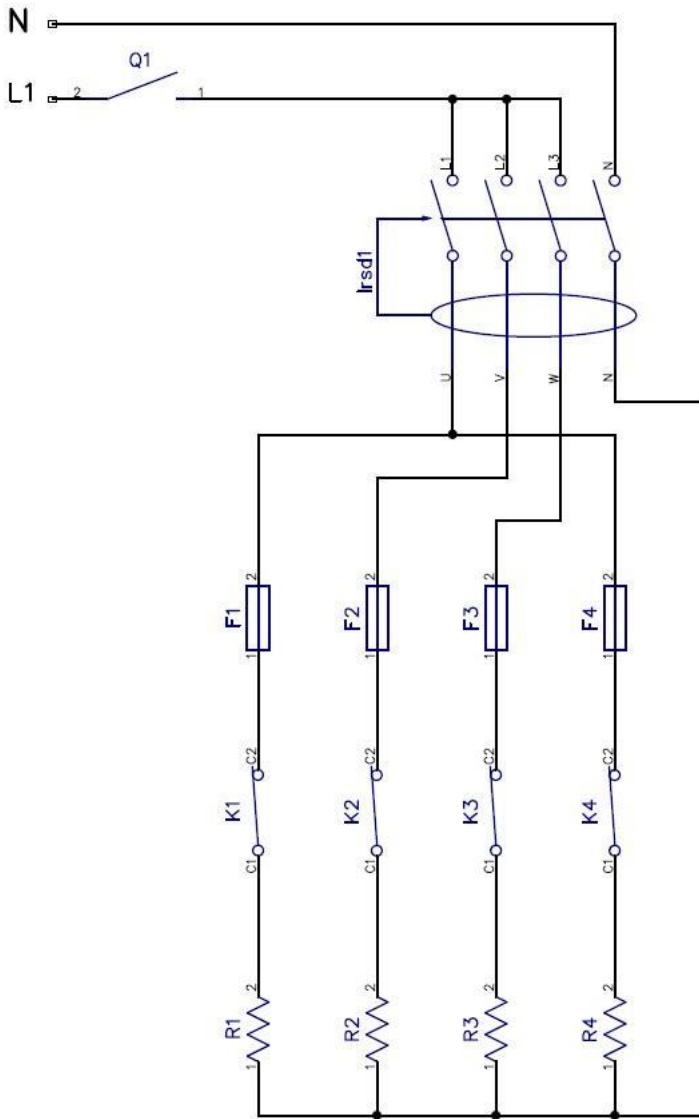
kuva 7. Keskuksen kytkentäkaavio
